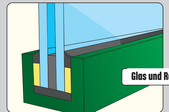
Vorlegeband Isolator und Abstandshalter zwischen Glas und Rahmen.
